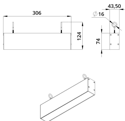
Габаритный чертеж
